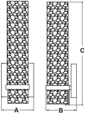
A: 4-1/4" B: 4" C: 13-1/2"
